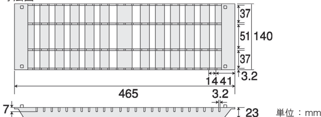
寸法図
