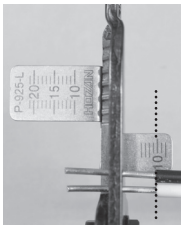
10mmに合わせる例
