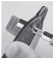
12mmに合わせる例
